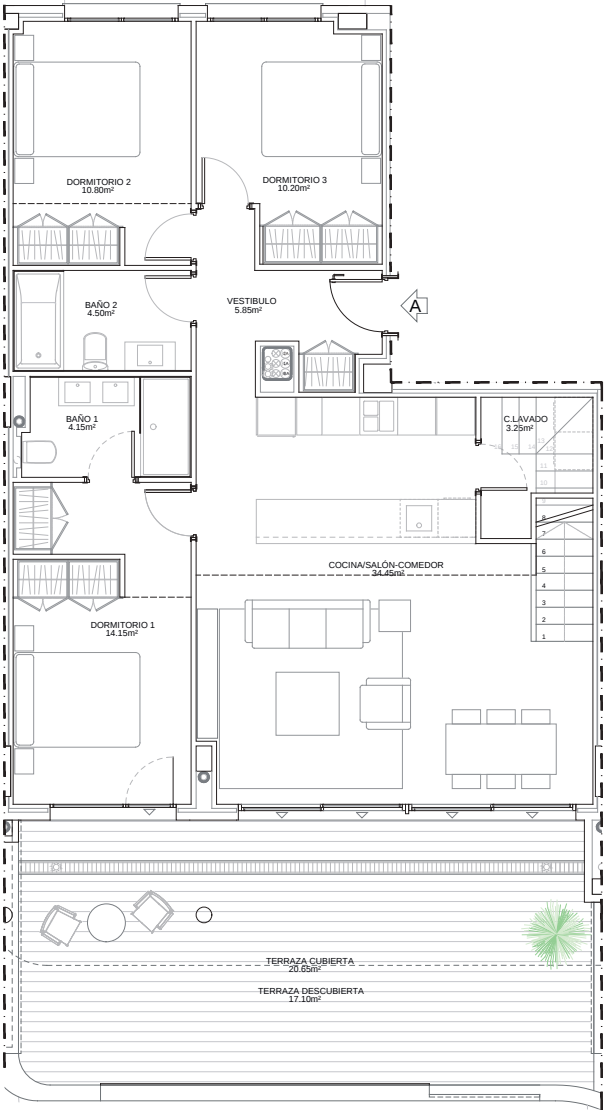
PLANTA 2ª
